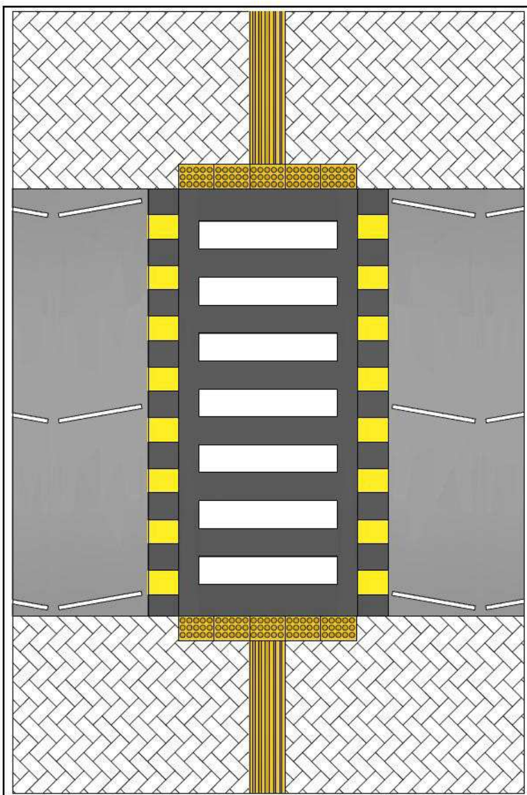
Figura 5-6 Attraversamento pedonale rialzato
