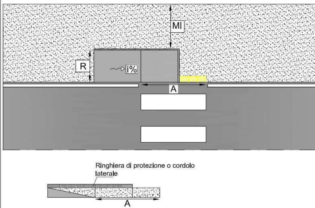
Figura 4-7 Rampa - schema 1c
