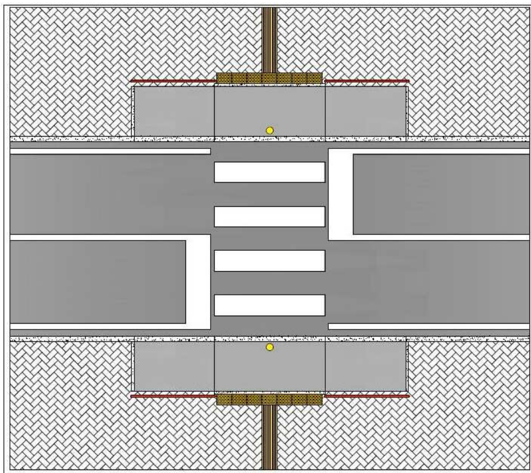
Figura 5-1 Attraversamento pedonale semaforizzato
