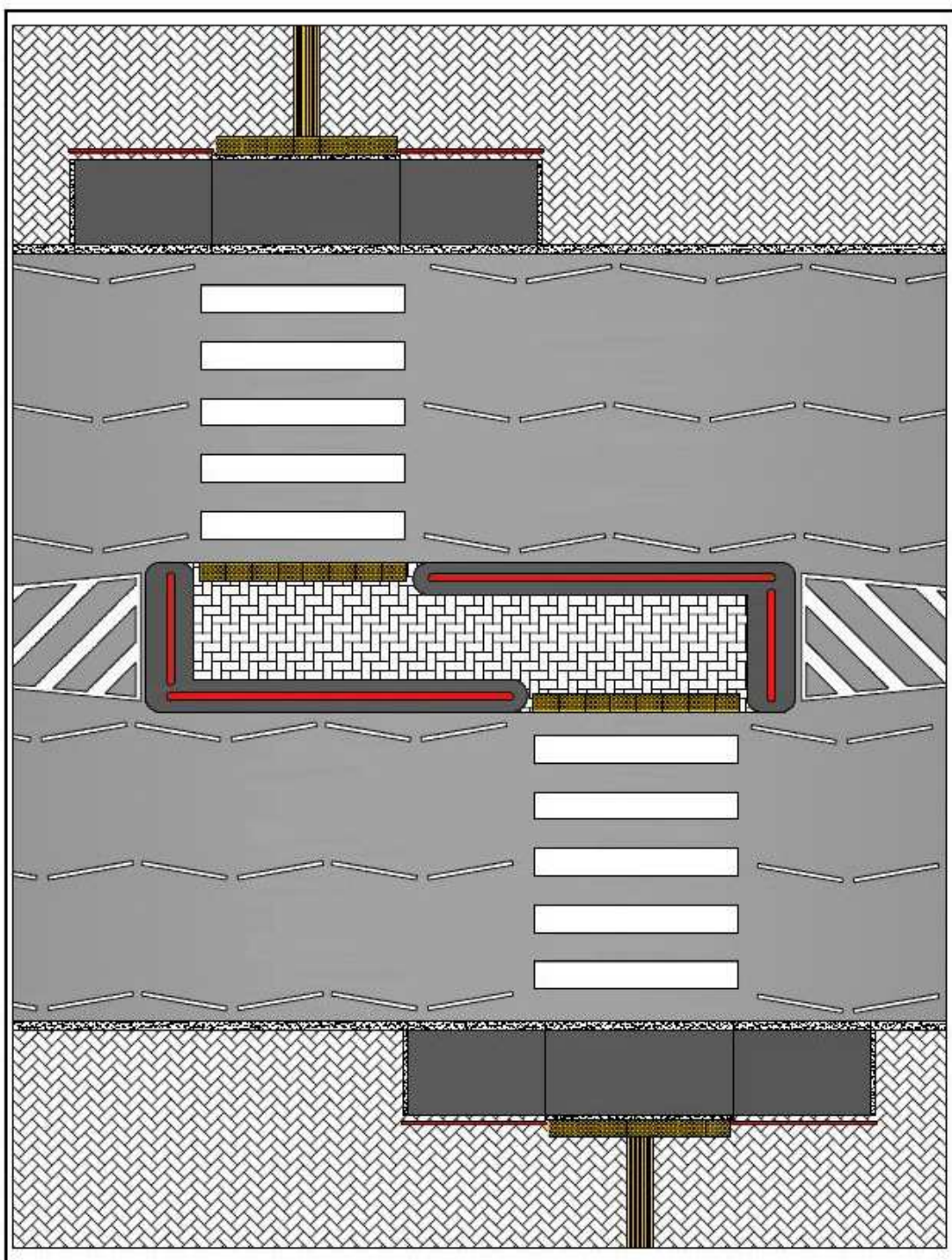
Figura 5-5 Attraversamento pedonale sfalsato
