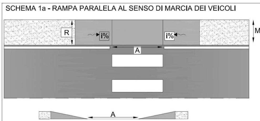
Figura 4-5 Rampa – schema 1a
