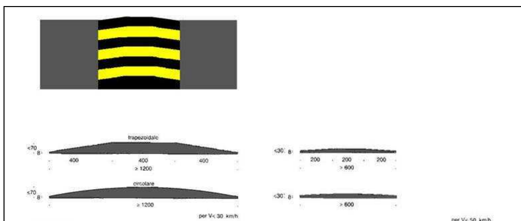
Figura 4-15 Dossi artificiali
