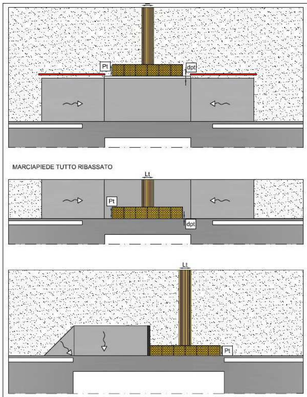
Figura 4-12 Pavimentazione tattile
