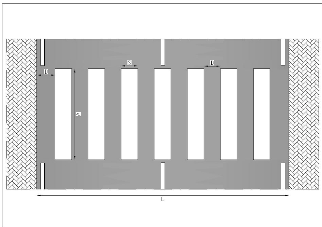
Figura 4-1 Attraversamento pedonale, le "ZEBRE"
