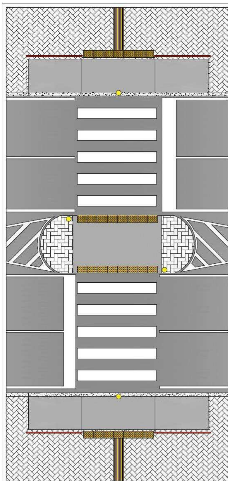
Figura 5-2 Attraversamento pedonale semaforizzato con isola salvagente
